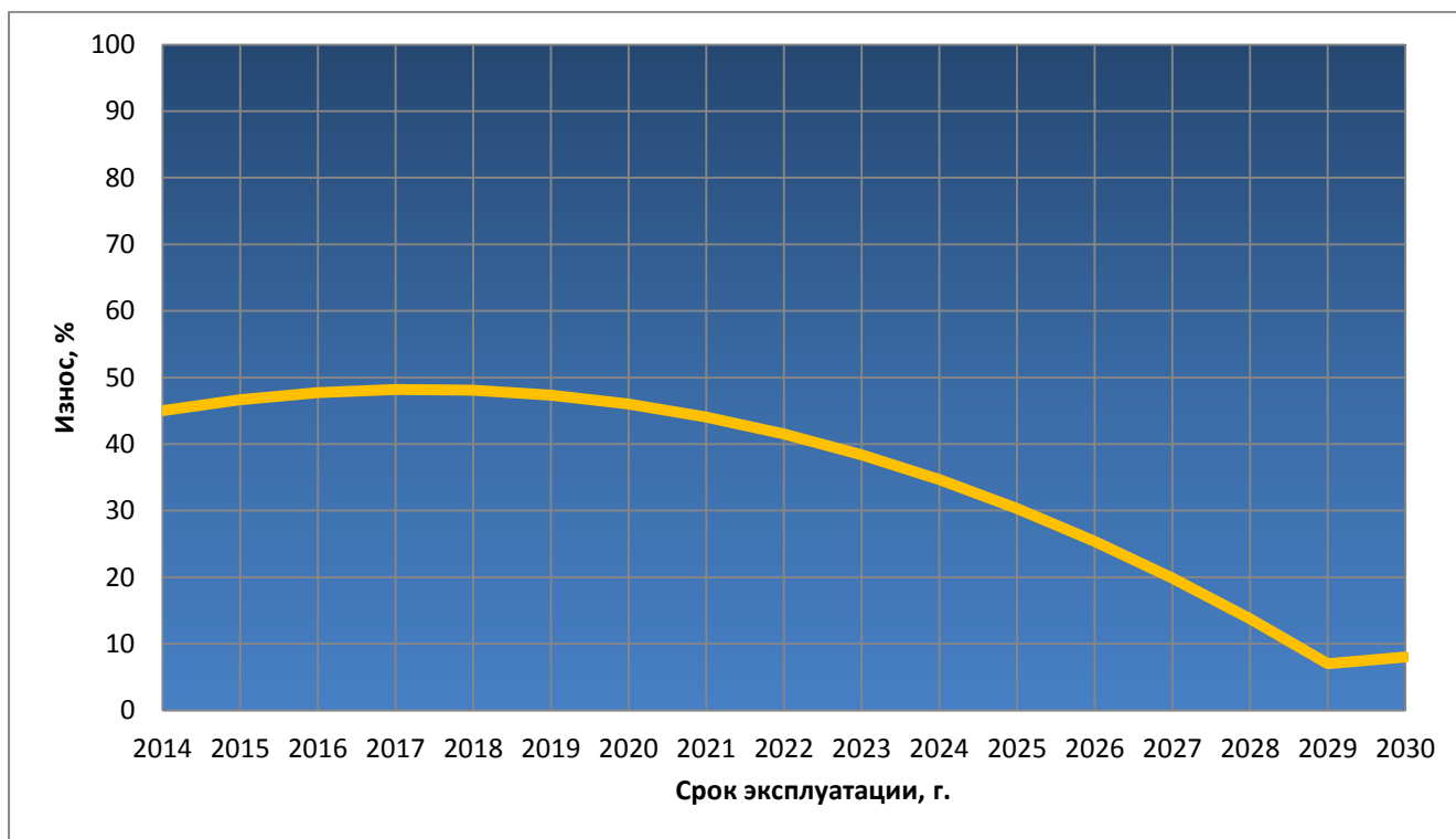
Рисунок 7.2 - Зависимость износа тепловых сетей от срока эксплуатации
